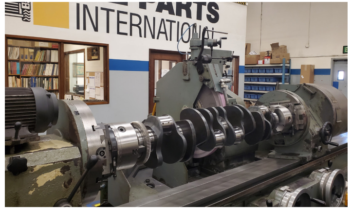
Configuración del cigüeñal para rectificar
